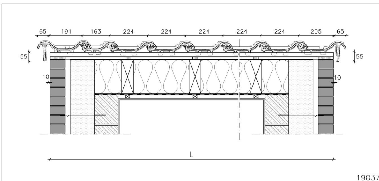
Fig.3: Breedteverdeling PREMION® pannen
