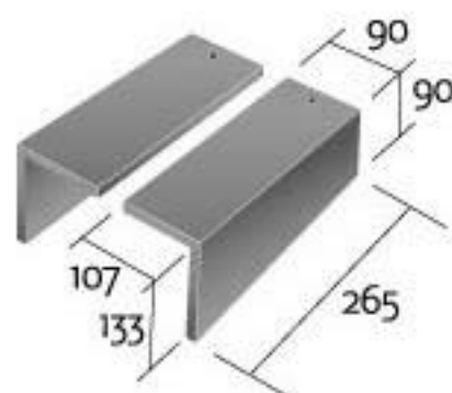
Gevelpanen links-rechts 1 gat Ø 5 mm
