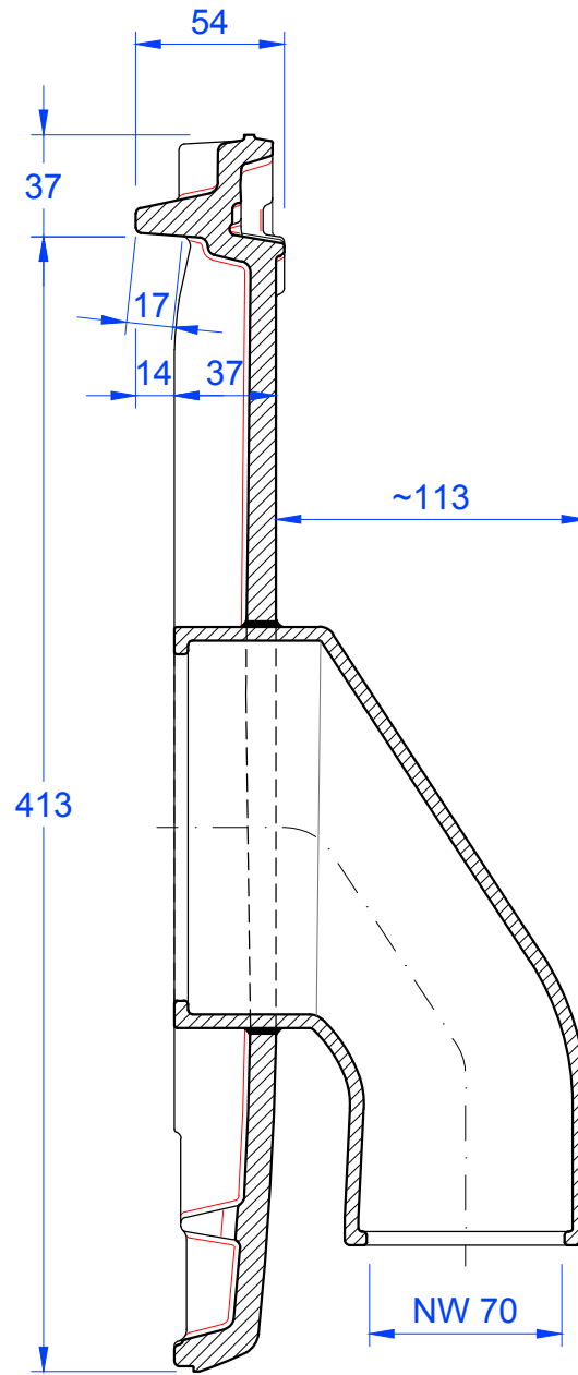
Schnitt B-B
