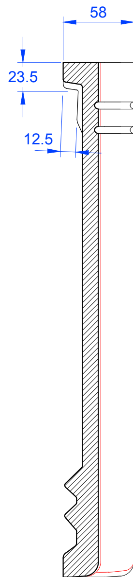
Schnitt B-B
