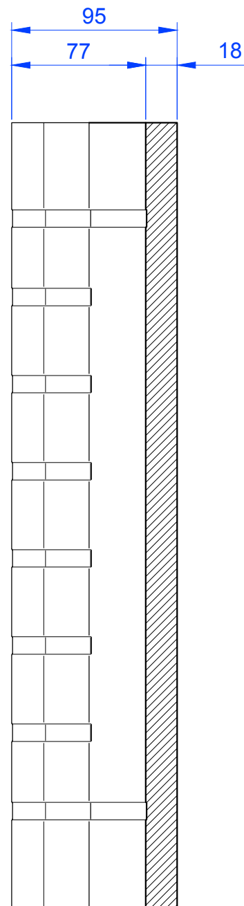
Schnitt A-A
