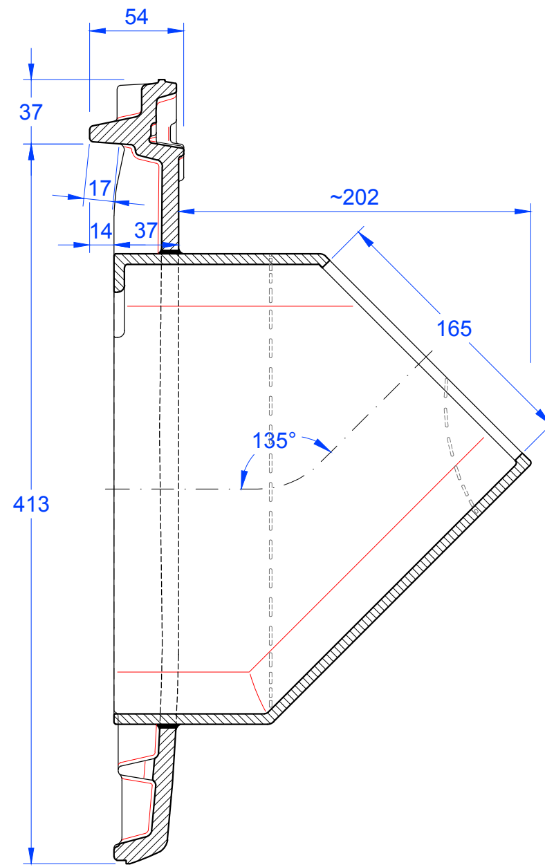
Schnitt B-B
